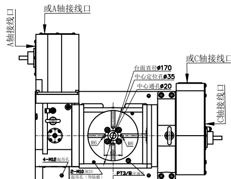
台面T型槽图
